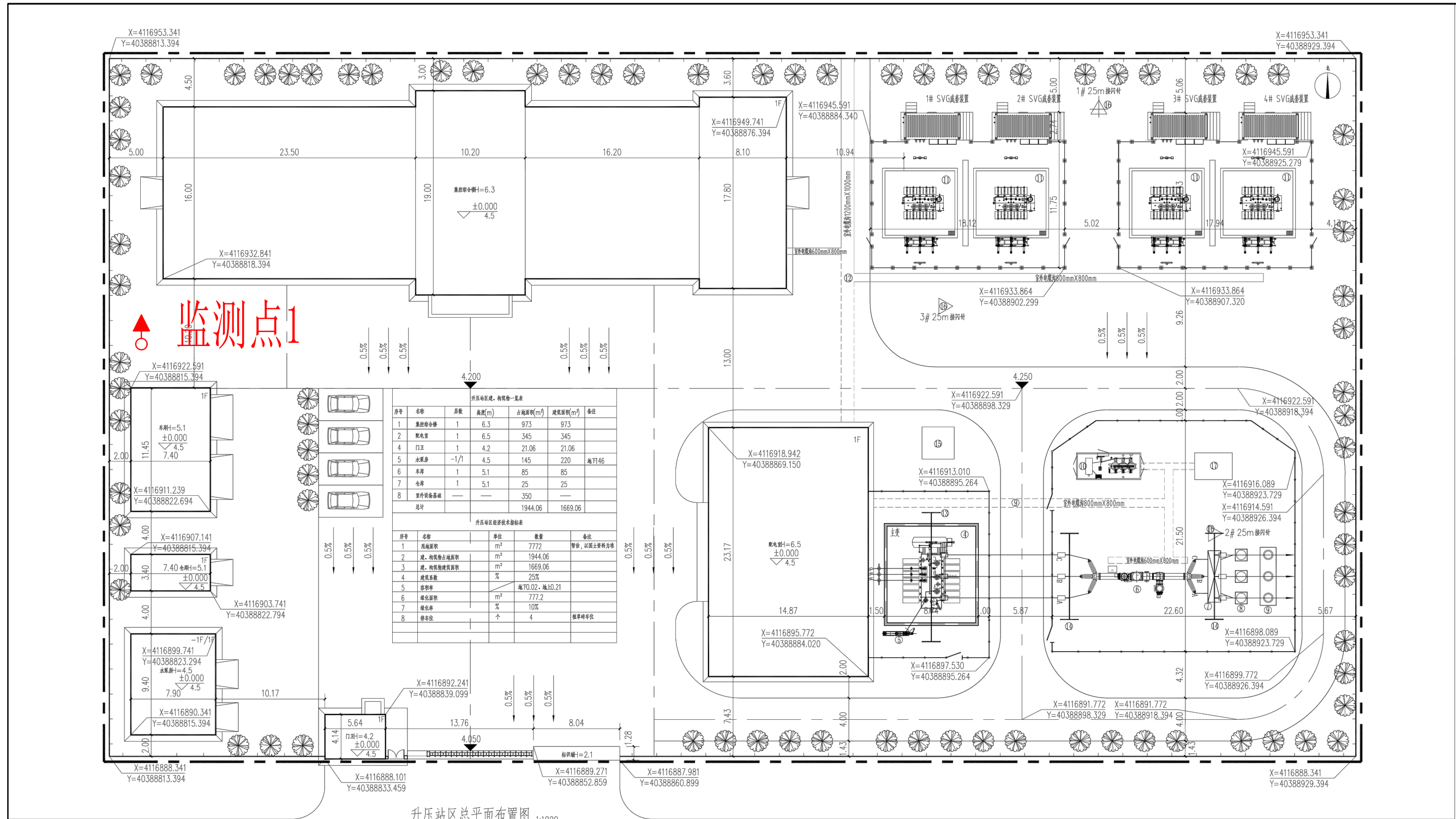
升压站总平面布置图 1:1000
