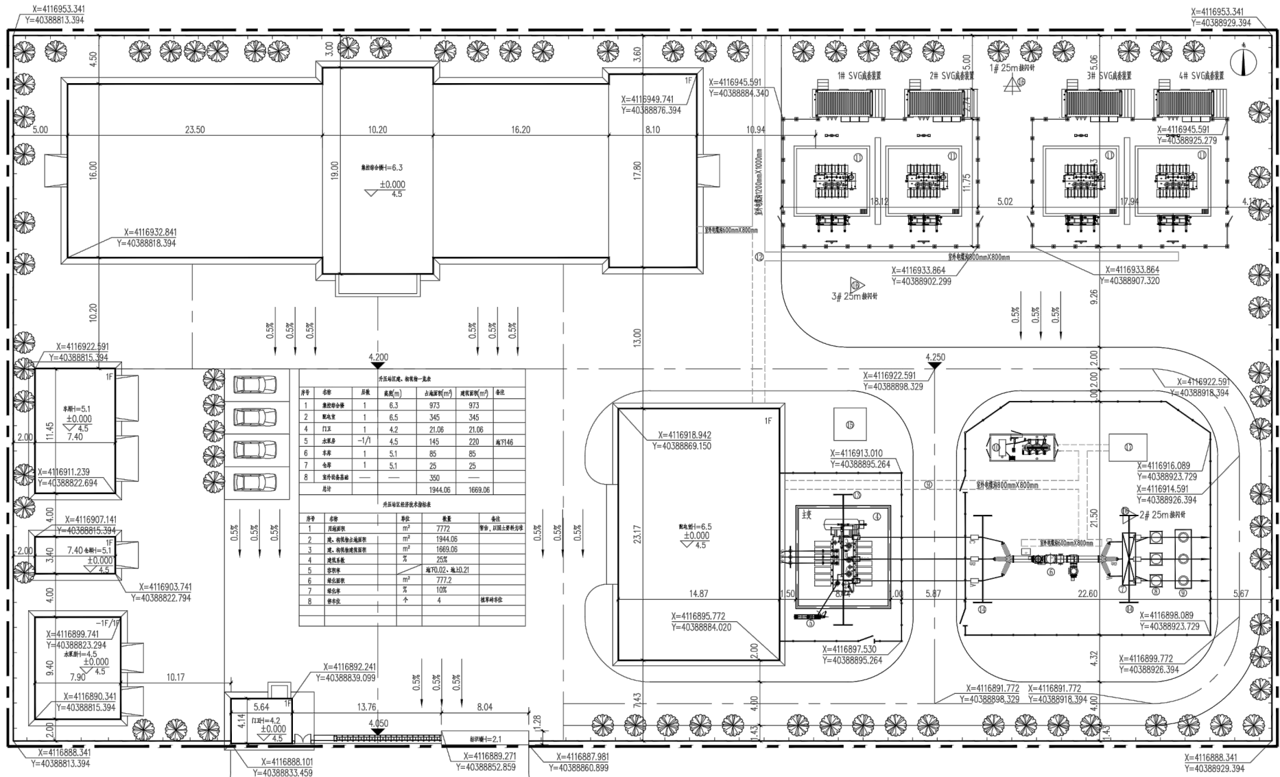
升压站区总平面布置图 1:1000
